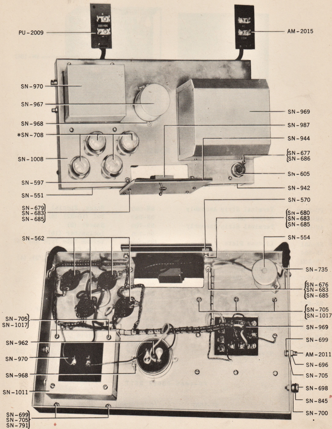
PU - 1003 POWER UNIT
