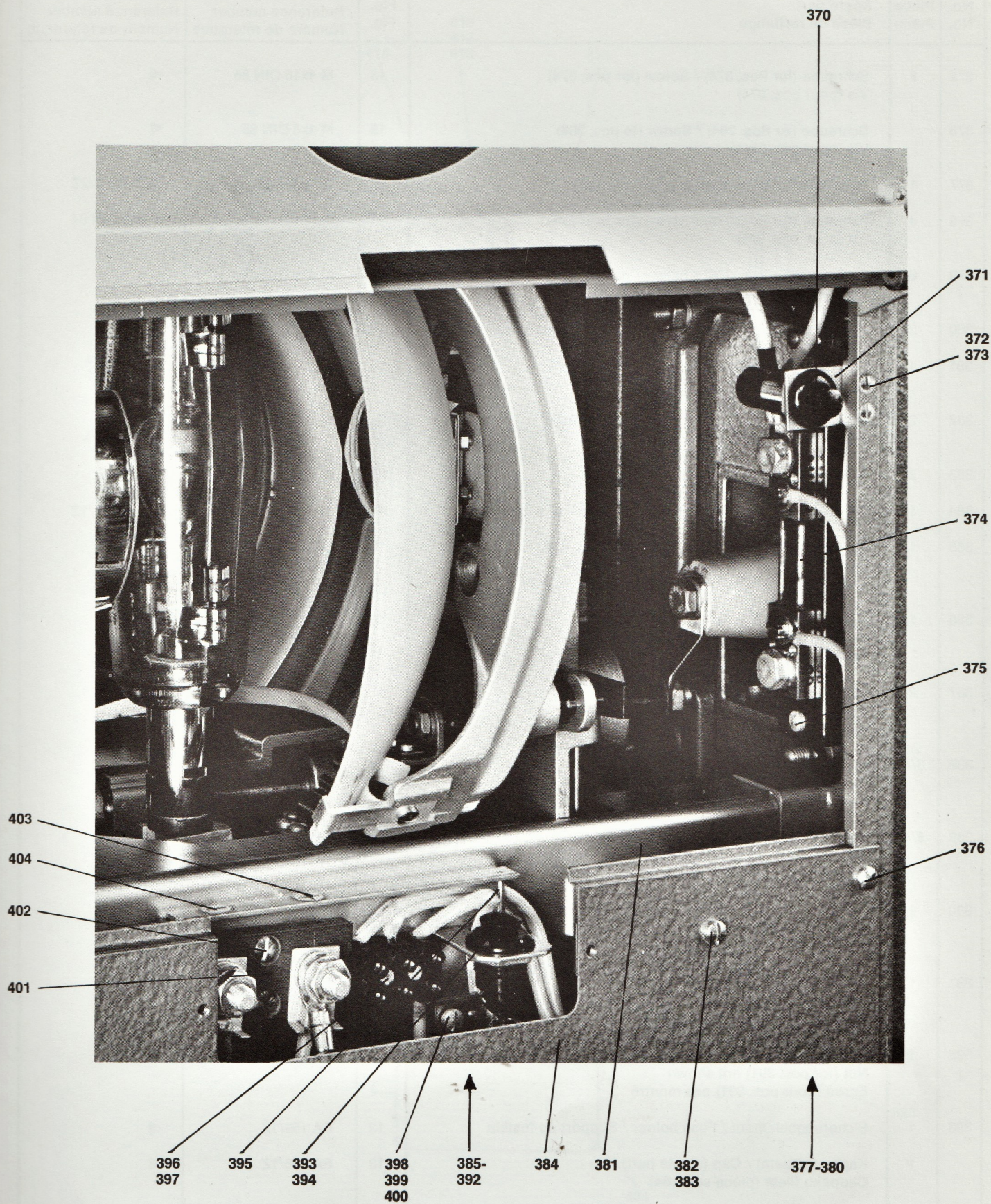
Xenonlampenhaus, Rückseite Xenonlamphouse, rear side Lampe au Xénon, vue arrière
